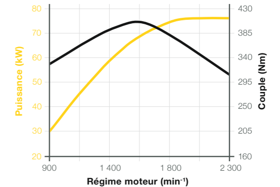
Courbe de puissance Deutz TCD 3.6, 74,4 kW, Euro V (en option)
