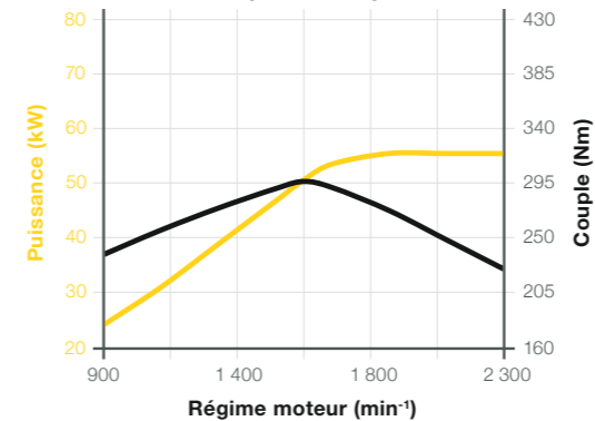
Courbe de puissance Deutz TCD 2.9, 55,4 kW, Euro V (standard)
