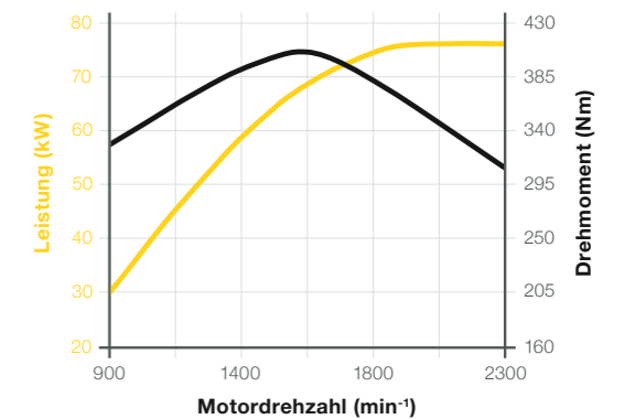
Leistungskurve Deutz TCD 3.6, 74,4 kW, Stufe V (Option)
