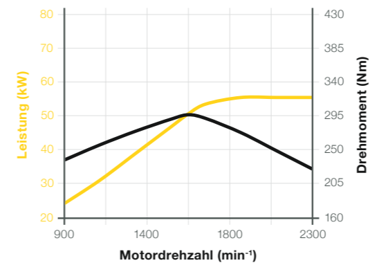
Leistungskurve Deutz TCD 2.9, 55,4 kW, Stufe V (Serie)
